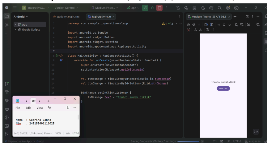
Project A - XML/View (Imperatif) (setelah di klik)
